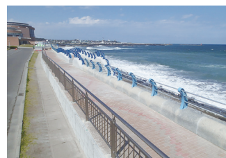
2. 海岸護岸改修(大洗町磯浜)
