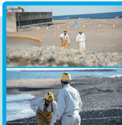
2. 海岸護岸改修(大洗町磯浜)
